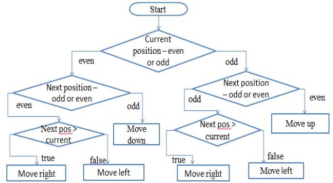
Fig.4. Flowchart
